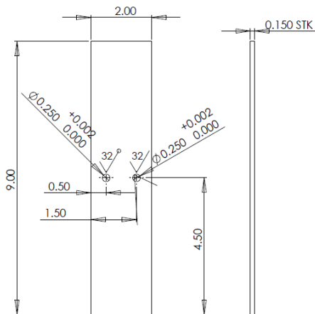
Fatigue test coupon
