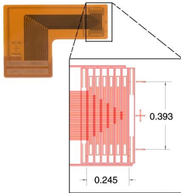
MWM-Array FA75
