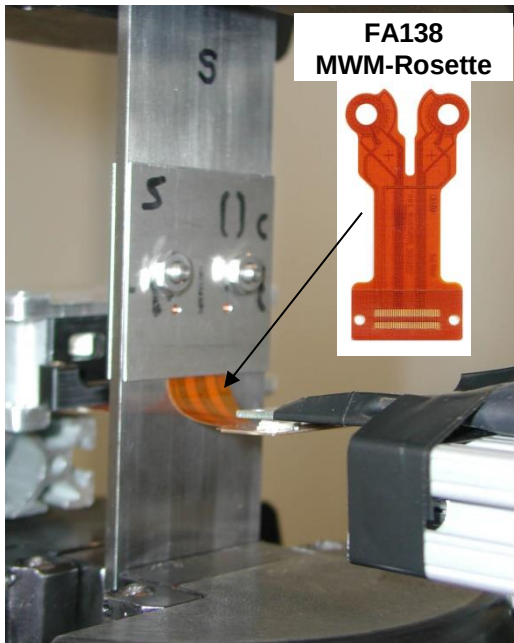
Fatigue test coupon
